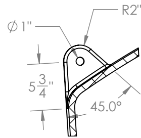
SECTION A-A SCALE 1 : 12
