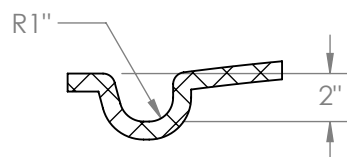
SECTION B-B SCALE 1 : 8
