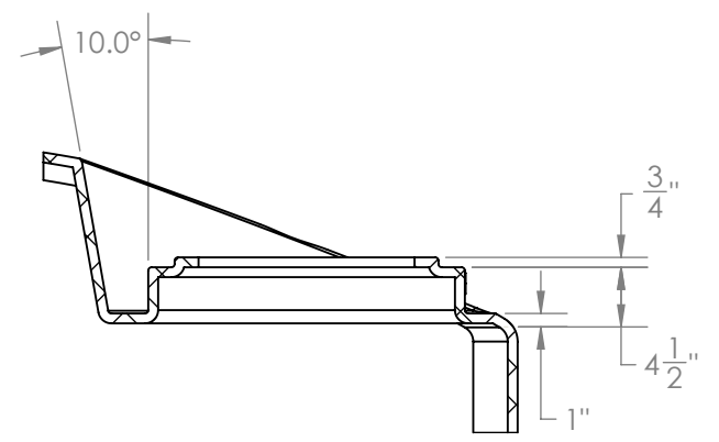
SECTION A-A SCALE 1:16
